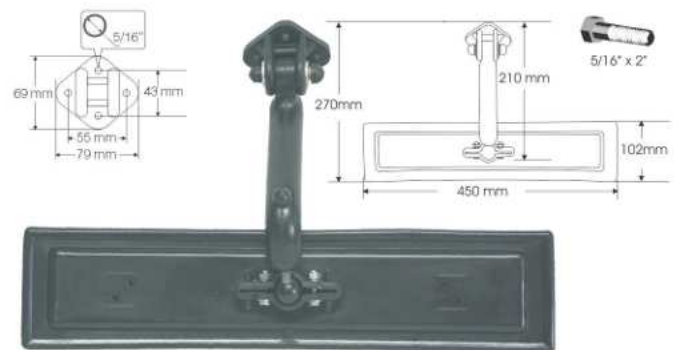
3-37 Espejo plástico, Luna Panorámica, soporte plástico Largo.
