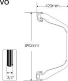
SOPORTE TIPO CAIO BUSES TRANSPORTE MASIVO
