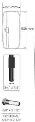
2-174L Espejo plástico. Con luz direccional.
