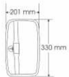
2-134-AP-S Espejo plástico.
